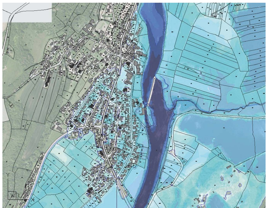
Hochwassersituation Münchshofen; aktueller IST-Zustand im Falle eines „HQ 100“ (Quelle: EBB Ingenieurgesellschaft mbH)
