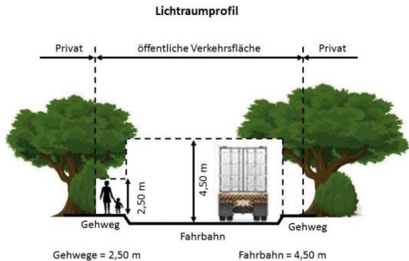
Grafische Darstellung des freizuhaltenden Licht- und Straßenverkehrsraums bei (Garten-)Bepflanzungen entlang Straßen. (Quelle: Gemeinde Wachtberg)
