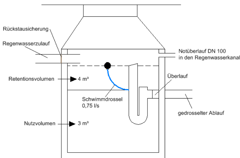
Abbildung 1 Schemaskizze Retentionsanlage
