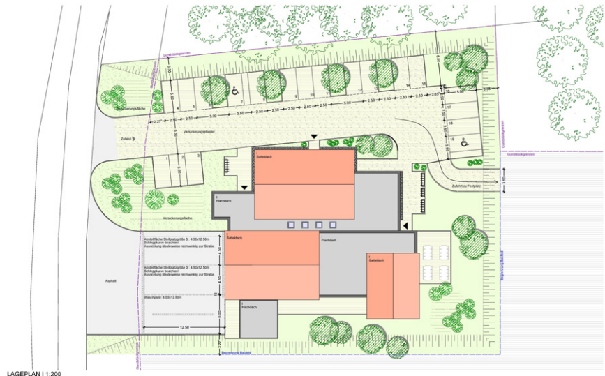
LAGEPLAN | 1:200
