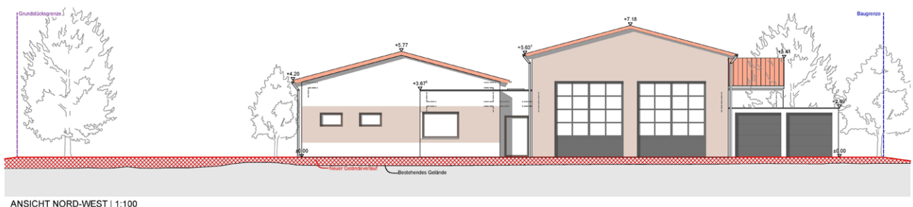
ANSICHT NORD-WEST | 1:100
